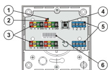
Figure 1: 1- Indicateur à LED jaune; 2- Indicateur à LED rouge; 3- Bornes du BUS; 4- Contact de sabotage avant; 5- Bornes auxiliaires; 6- Code Mémoire
